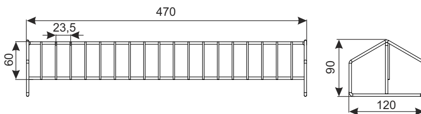
Przegroda poprzeczna drucziana L-470
