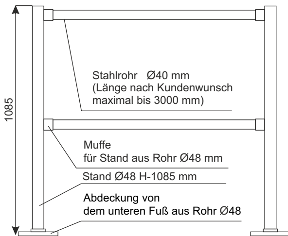
RAUMTEILER H-1085 mm:
