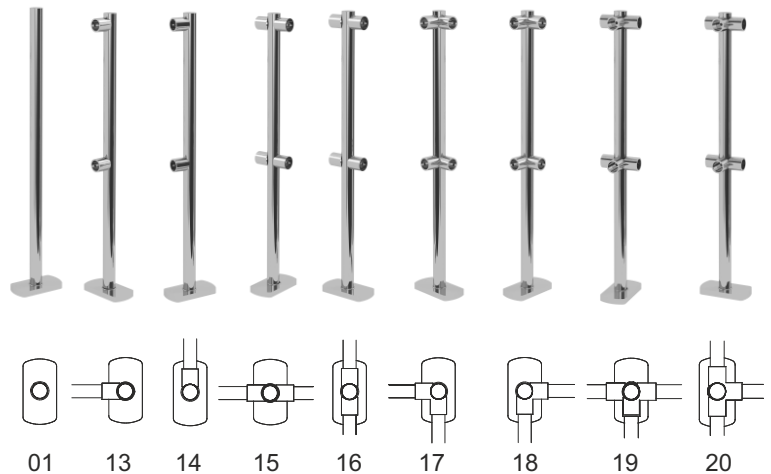
KOMPLETTER STAND H-1085 (Ständer mit unterer Fußabdeckung und Muffen) - KONFIGURATIONEN:
