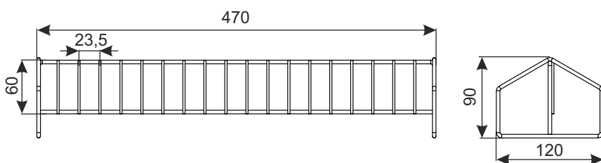
Drahtquertrennwand L-470
